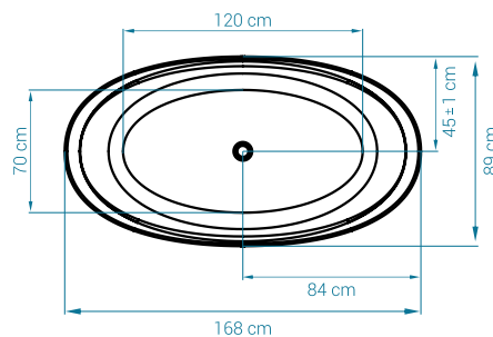
Vista Superior
