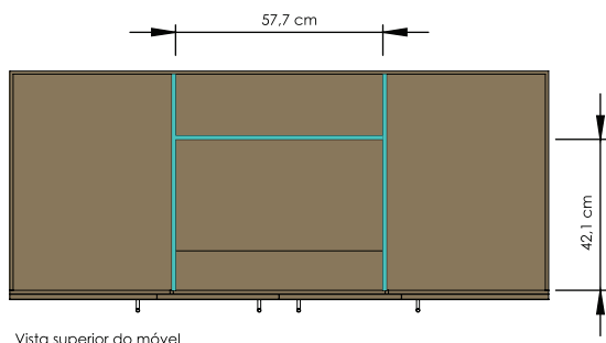
Vista superior do móvel
